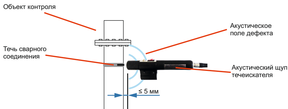
Рис. 7. Схема поведения контроля герметичности способом УЗ-щупа течеискательного комплекса «ТИ1-ЗОНД+»
